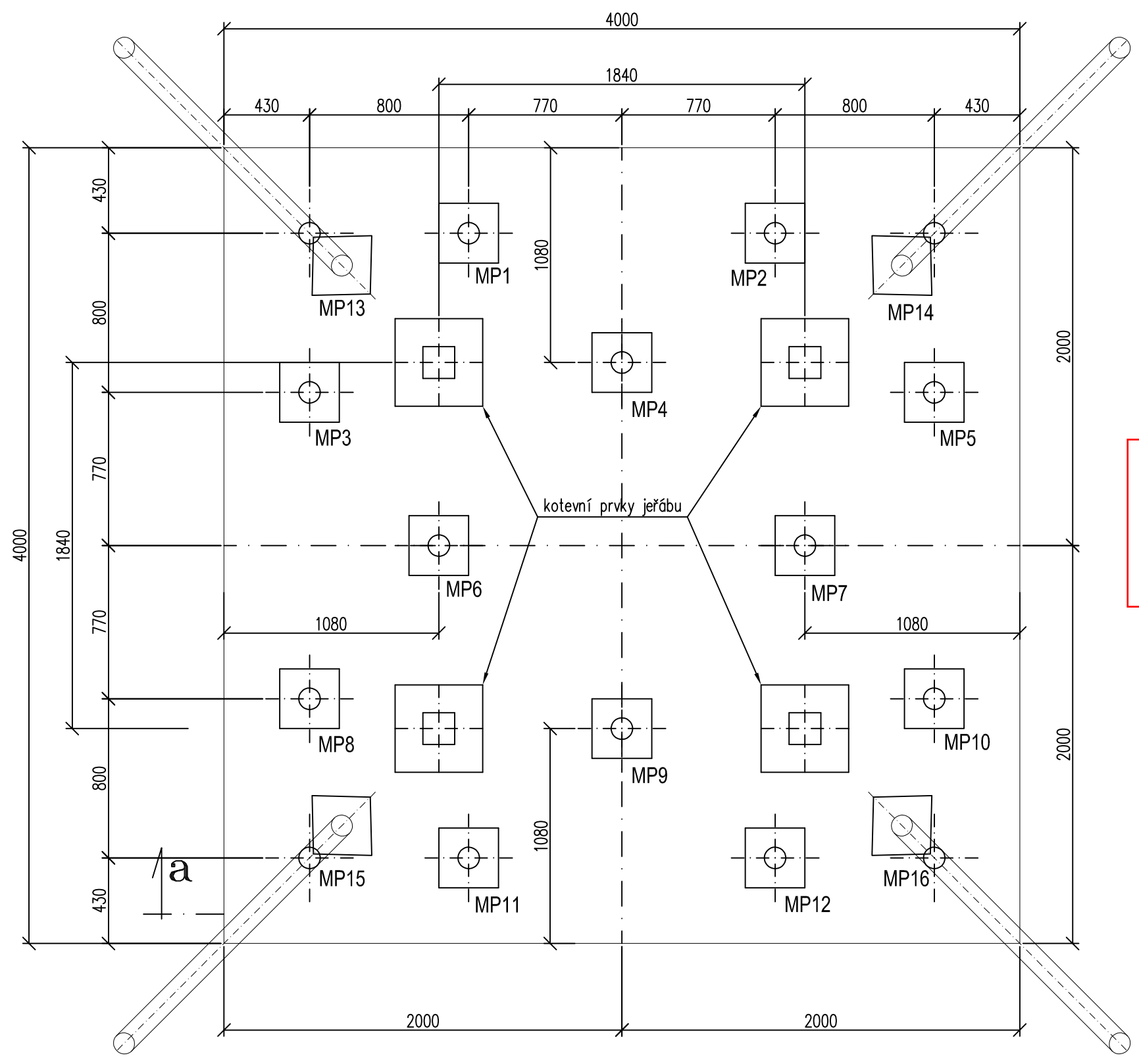
Půdorys s rozměry a popisem mikropilot
