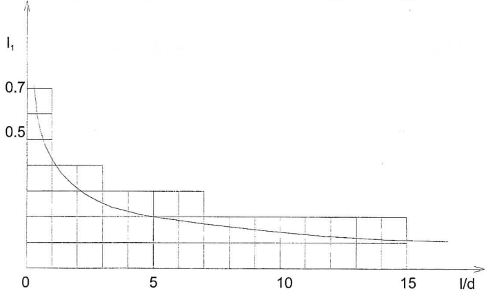
Obr. 20 Příkladový koeficient sedání I_1
