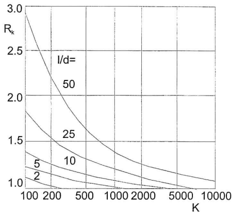
Obr. 21 Korekční součinitel R_k
